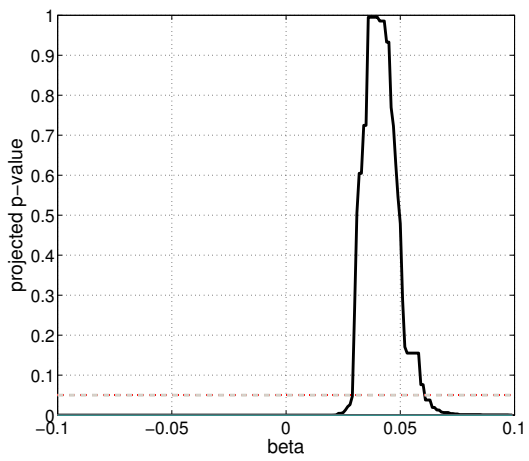
(d) Basic equation: 1940-50: projected p -value
